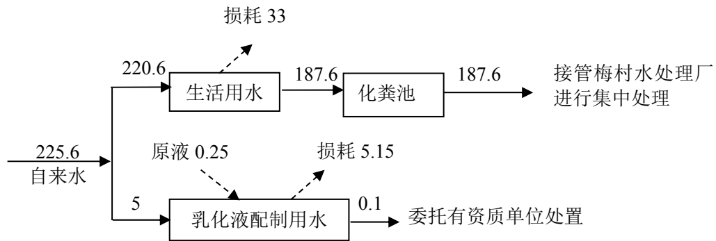
图 2-1 实际水平衡图 (单位: t/a)
