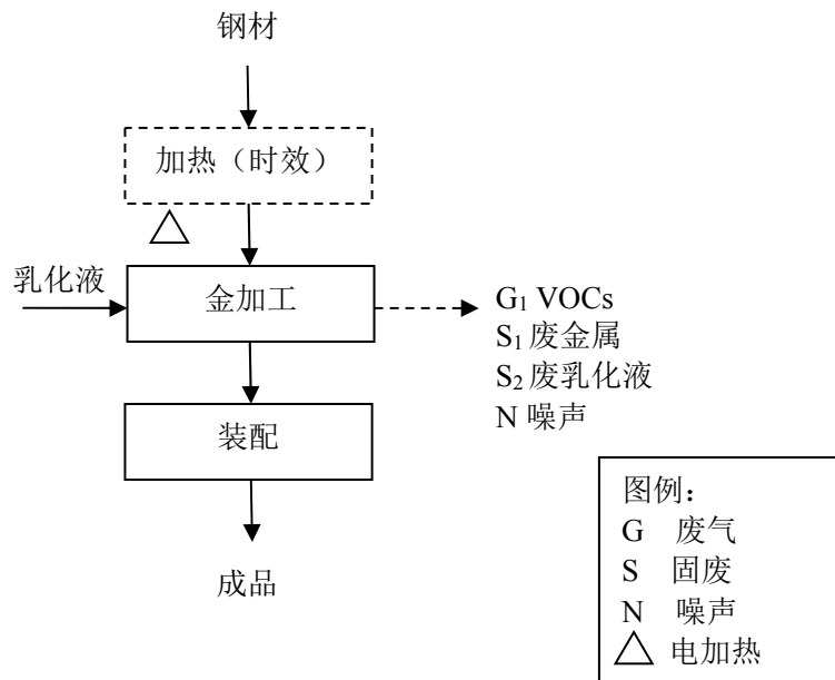
图 2-2 非标检验夹具生产工艺流程图
